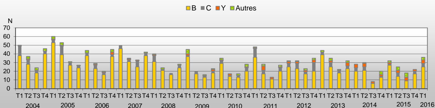
Méningococcémies en Belgique par trimestre : 2004-2016
